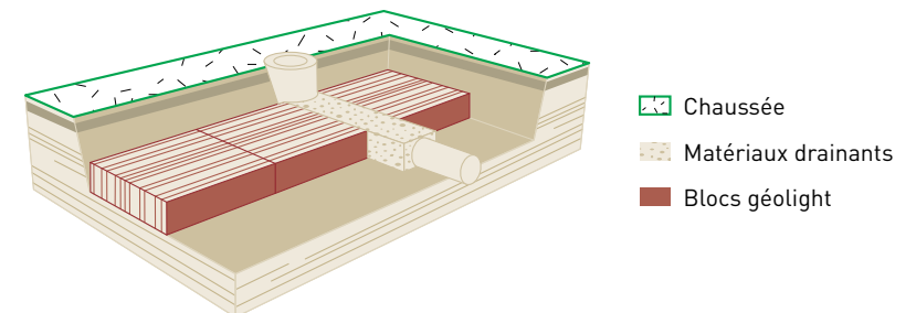
PRINCIPE DE FONCTIONNEMENT D'UNE STRUCTURE GÉOLIGHT
