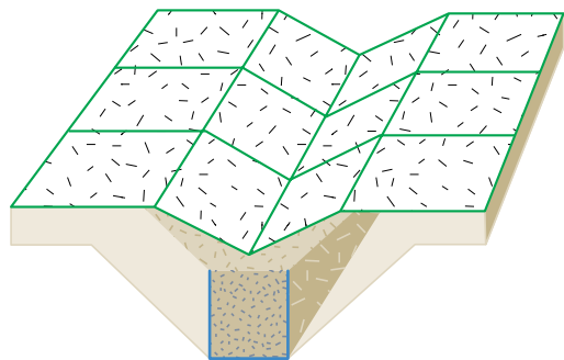
NOUE AVEC MASSIF DRAINANT
