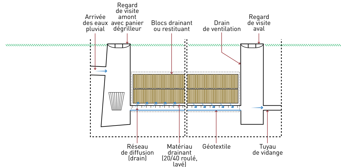
PRINCIPE DE FONCTIONNEMENT D'UNE STRUCTURE GÉOLIGHT
