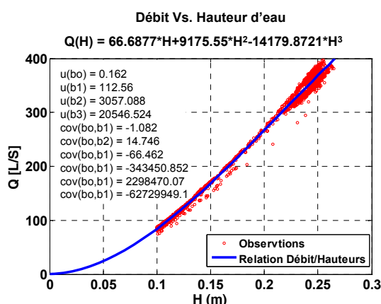
Figure 2-5. Régressions polynomiales au sens de Williamson de la relation Débit/Hauteurs .
