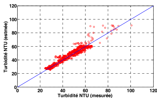
Figure 2-11. Comparaison entre la turbidité mesurée réelle et celle calculée avec la régression polynomiale.
