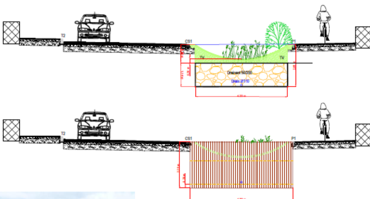
Coupe type d'une noue
