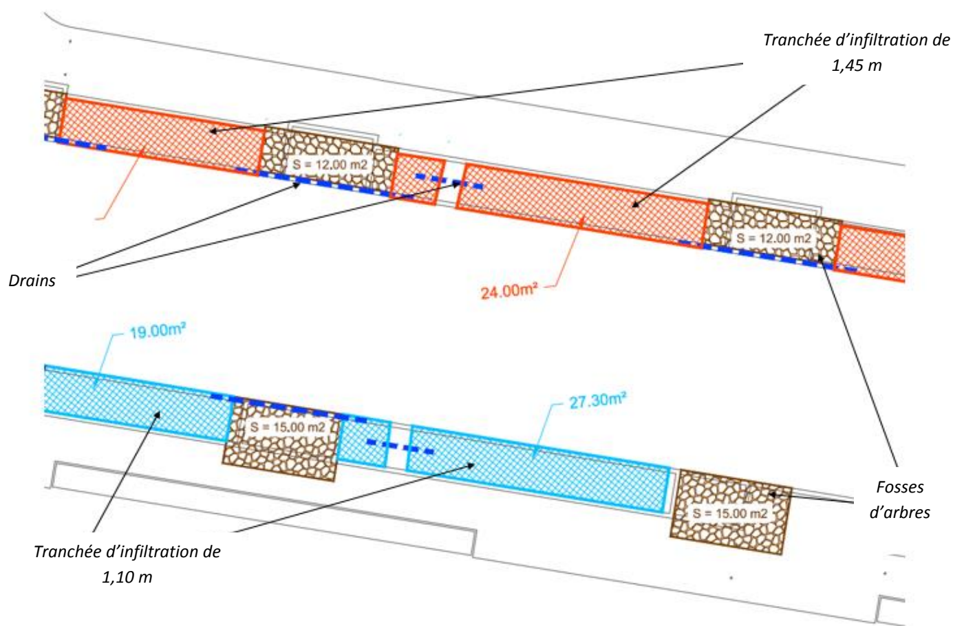
Vue en plan du principe de fonctionnement de l'infiltration sous le stationnement
