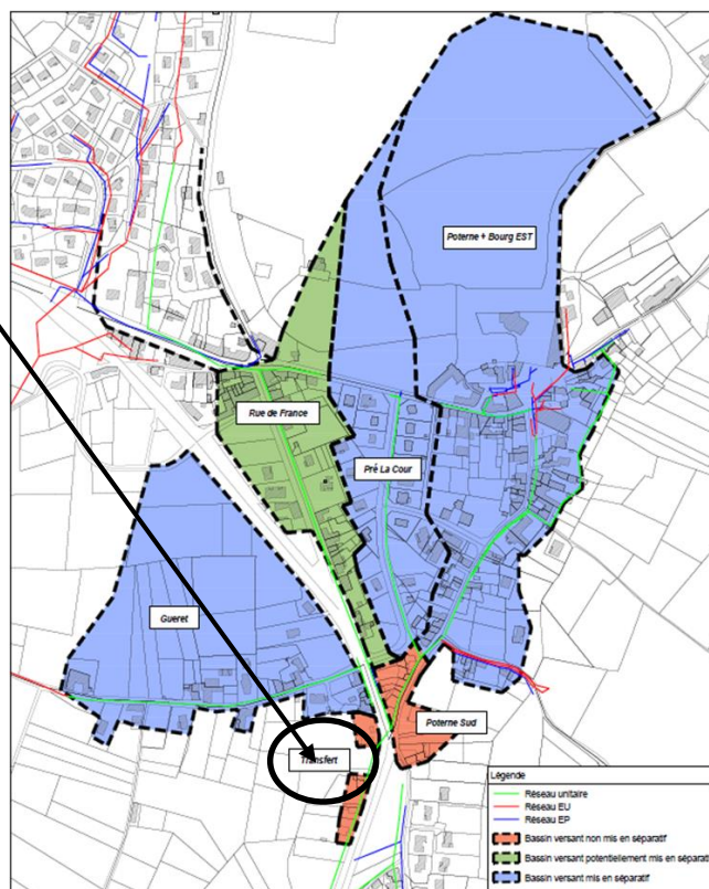
Surface active de raccordement à l'ouvrage
