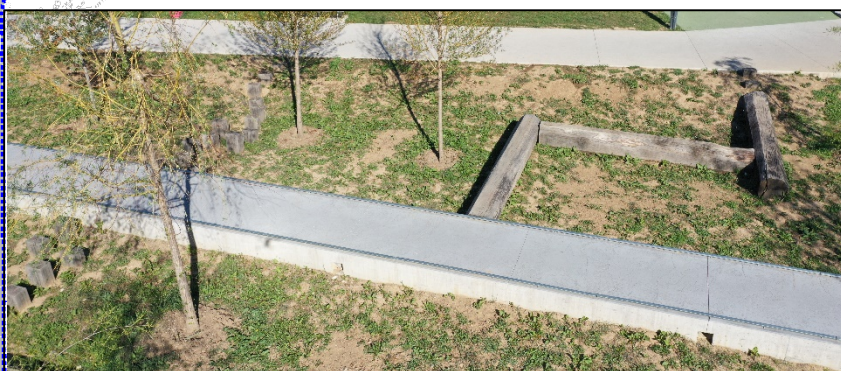
Photos du jardin de pluie
