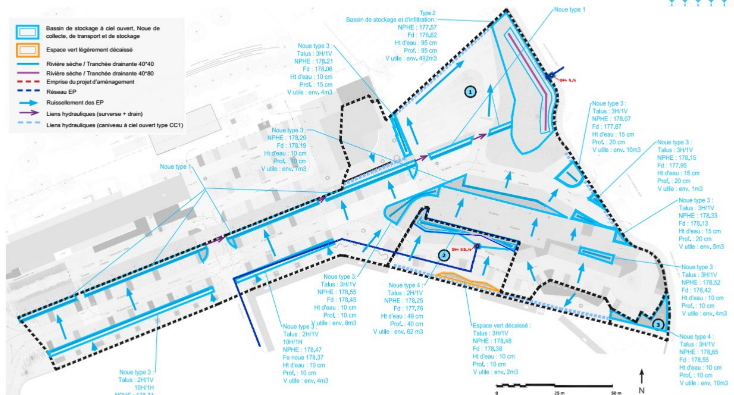
Schéma de gestion des eaux pluviales
