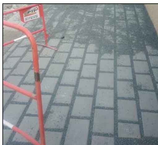
Phase travaux : réalisation de la couche de granulat stockant (à gauche) et pavés drainants (à droite)
