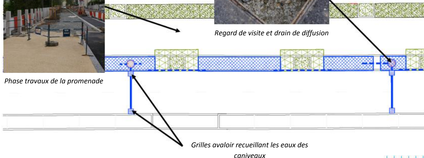
Vue de dessus du fonctionnement général du système
