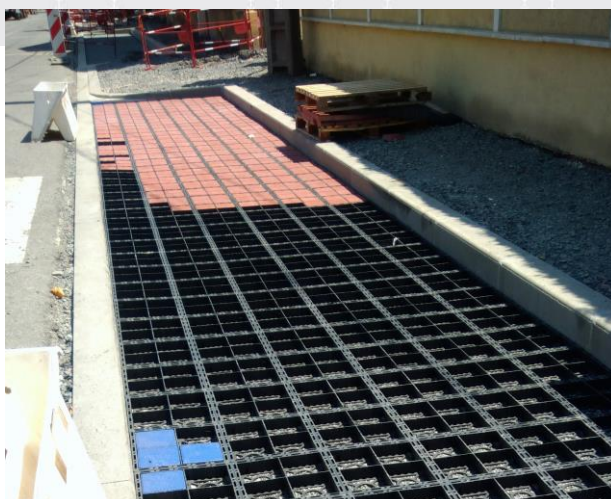
Pose des dalles alvéolaires et des pavés sur les places de stationnement
