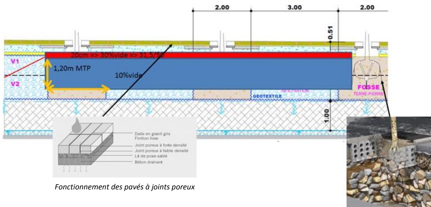
Coupe transversale détaillant le fonctionnement de la place de Francfort
