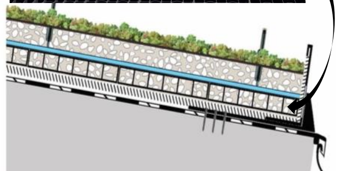
Système d'arrosage par aspersion et dalles alvéolaires pour pente forte
