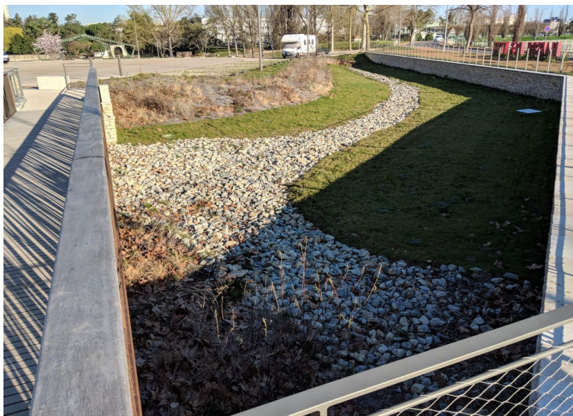
Photo d'un bassin sec, exutoire des tranchées drainantes
