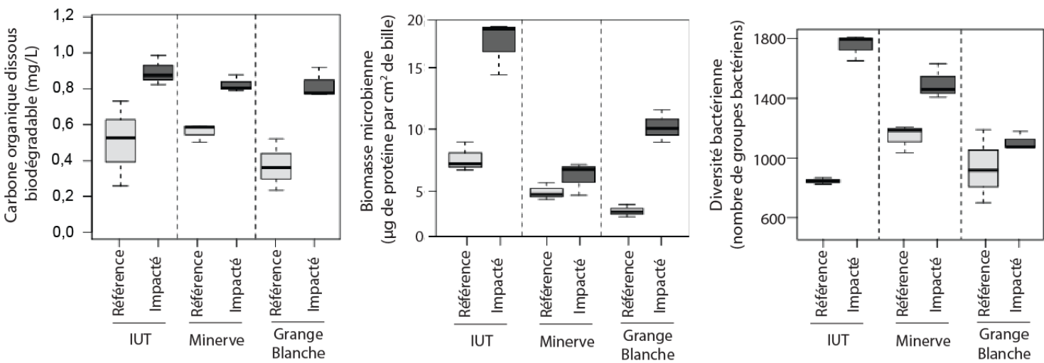
Fig. 36. Teneurs moyennes en carbone organique dissous, biomasse et diversité microbiennes en amont (référéce) et en aval (impacté) de trois bassins d’infiltration d’eau pluviale de la Métropole de Lyon (Voisin et al. 2020 dans Environmental Science and Pollution Research)
