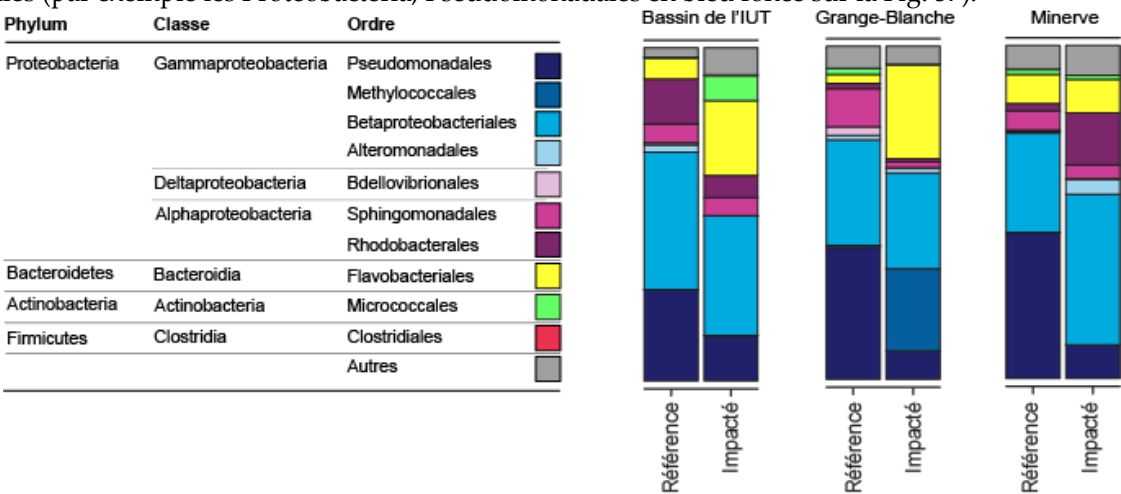
Fig. 37. Composition des communautés microbiennes en amont (référéce) et en aval (impacté) de trois sites d’infiltration de l’Est Lyonnais. Les différents taxons sont représentés en % du nombre de séquences (Lebon et al. 2021 dans Science of the Total Environment).
