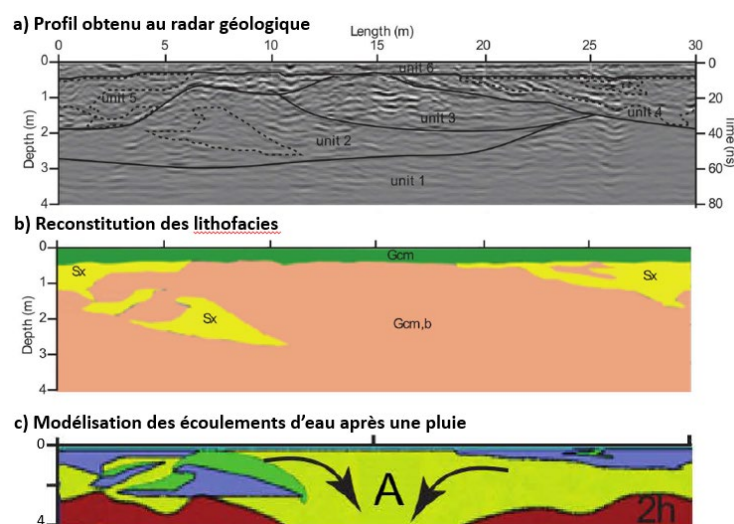
Fig. 19. Utilisation du radar géologique pour reconstituer les lithofacies présents sous un bassin d'infiltration et les chemins préférentiels de l'eau après une pluie (Coutinho et al. 2015)
